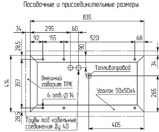
ТРК серии ПКИ 2.х.х. НСХ (напорная система)
